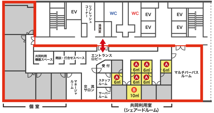
福島駅西口インキュベートルーム平面図
